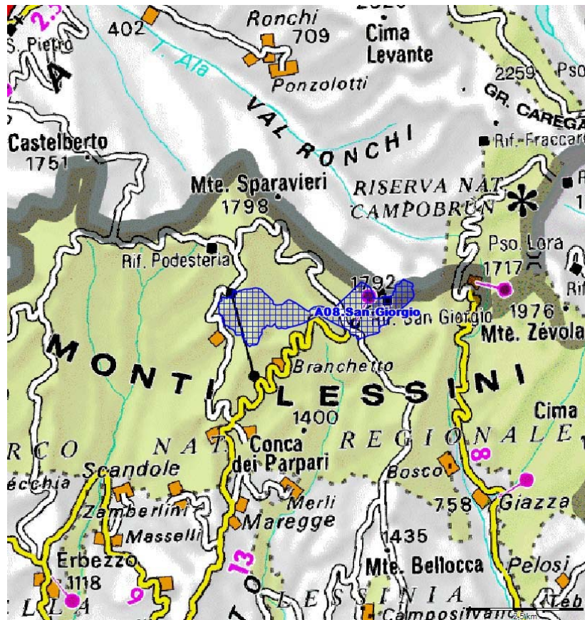
Fig. 1: Individuazione dell'ambito sciabile A08 San Giorgio rappresentato dal poligono campito di colore blu.
