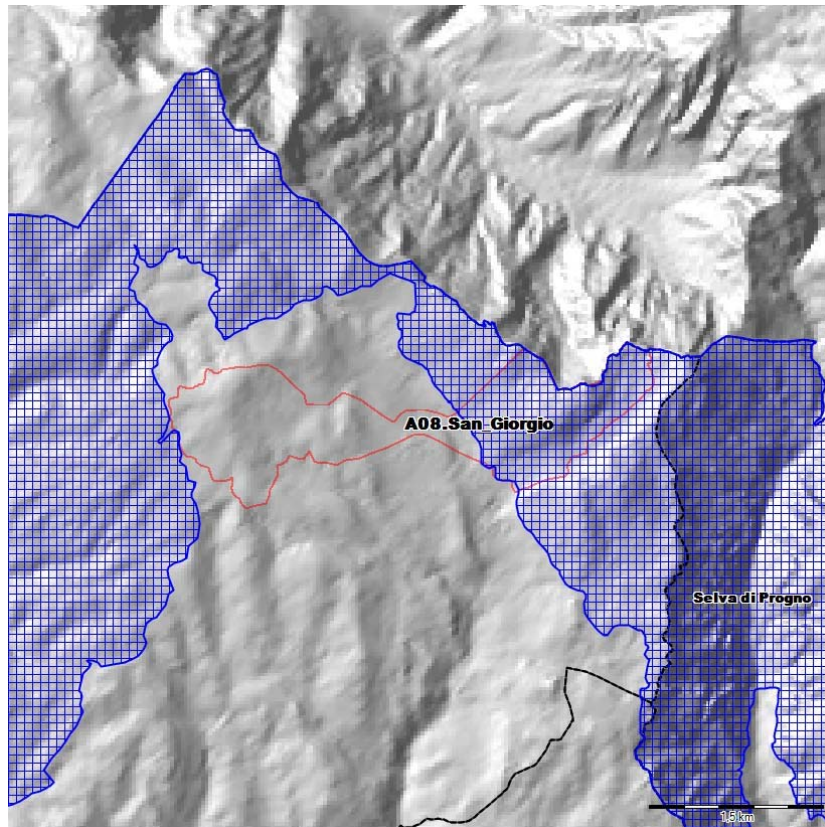
Fig. 4: Individuazione dell'ambito sciabile A08 San Giorgio rappresentato dal poligono di colore rosso. L'area evidenziata dalla campitura blu rappresenta il sito Natura 2000 coinvolto SIC- ZPS IT3210040. La linea tratteggiata di colore nero individua il confine amministrativo.
