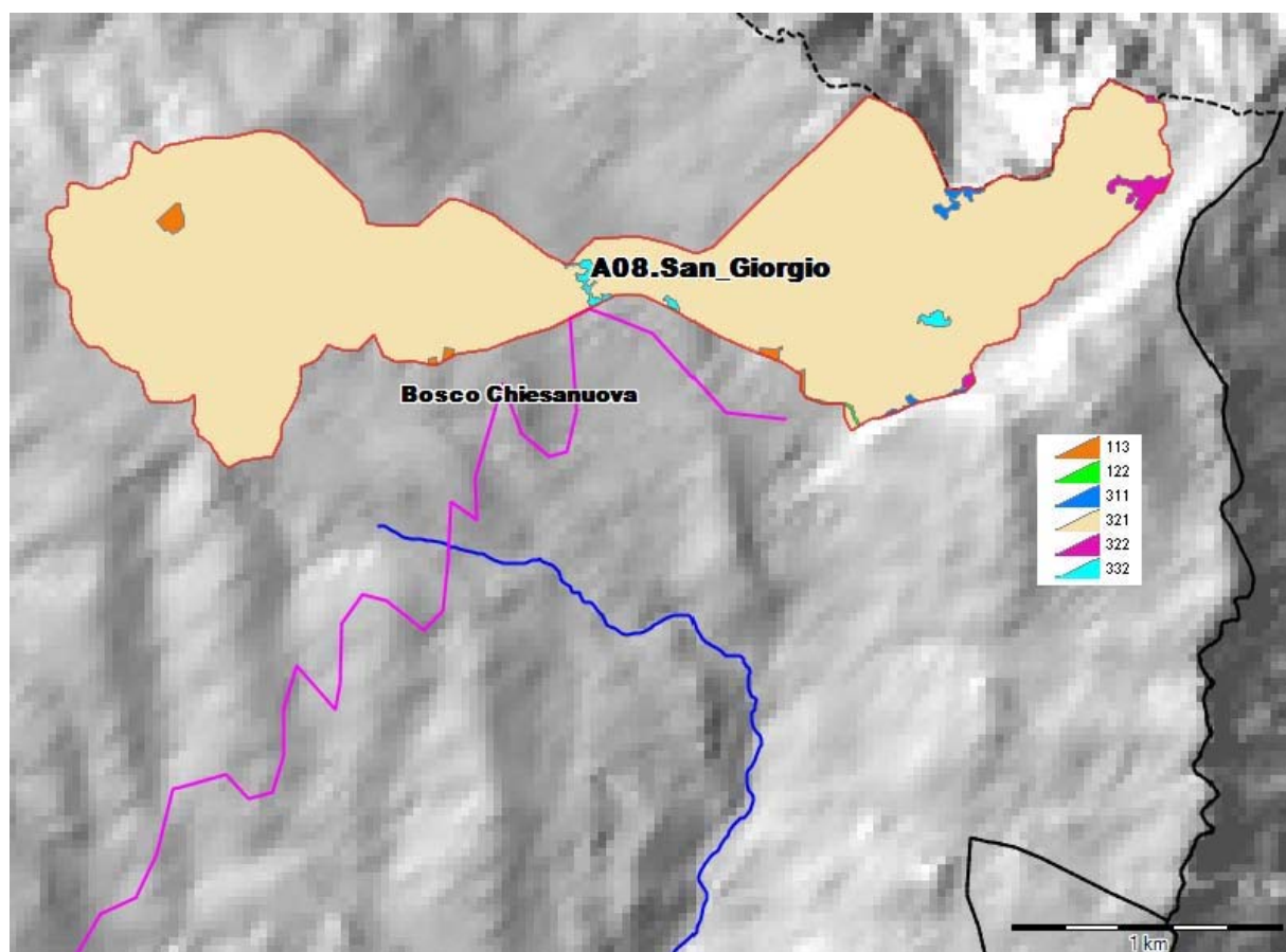
Fig. 6: Tipologie di copertura del suolo presenti nell'ambito sciistico A08 San Giorgio. Nell'immagine, in basso a destra, si riporta la legenda dei colori con i quali si evidenziano le tipologie di copertura del suolo, mentre la linea di colore rosso rappresenta il perimetro dell'ambito sciistico A08 San Giorgio, la linea di colore magenta rappresenta la viabilità principale, la linea di colore blu individua la rete idrografica e la linea tratteggiata di colore nero individua il confine amministrativo.
