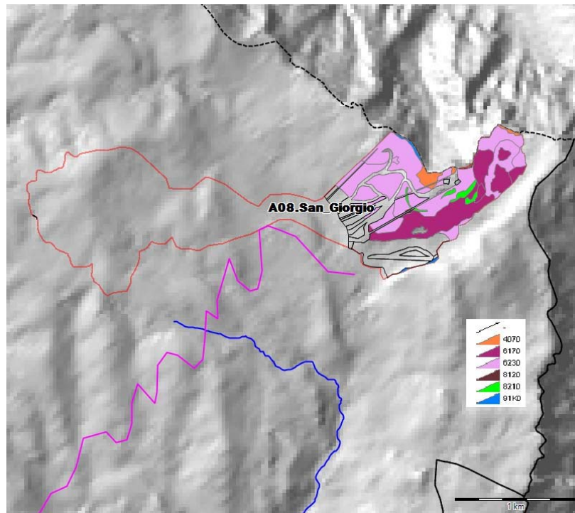
Fig. 5: Habitat comunitari coinvolti dall'ambito sciistico A08 San Giorgio. Nell'immagine, in basso a destra, si riporta la legenda dei colori con i quali si evidenziano gli habitat comunitari coinvolti, mentre la linea di colore arancione rappresenta il perimetro dell'ambito sciistico A08 San Giorgio, la linea di colore magenta rappresenta la viabilità principale, la linea di colore blu individua la rete idrografica e la linea tratteggiata di colore nero individua il confine amministrativo.
