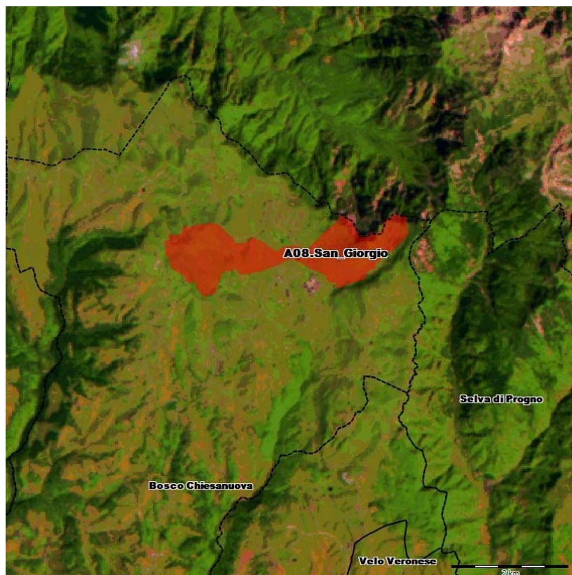
Fig. 3: Individuazione dell'ambito sciabile A08 San Giorgio rappresentato dal poligono di colore rosso. La linea tratteggiata di colore nero individua il confine amministrativo.
