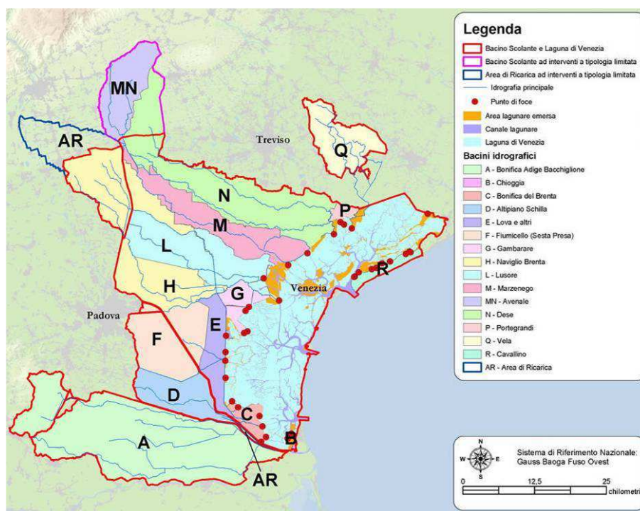
Figura: Bacini idrografici principali scolanti nella laguna di Venezia
