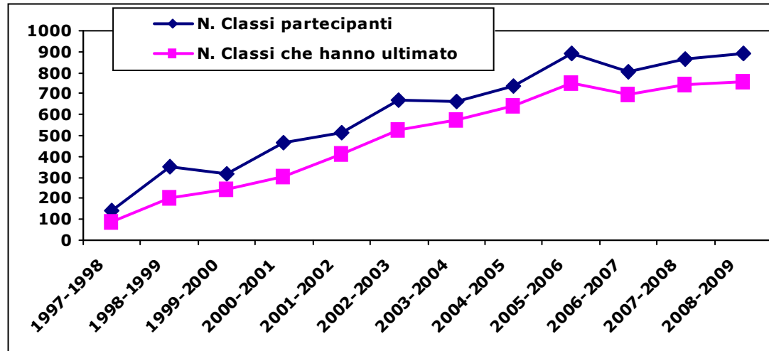
Fig.1 : Distribuzione assoluta classi partecipanti e che hanno ultimato
